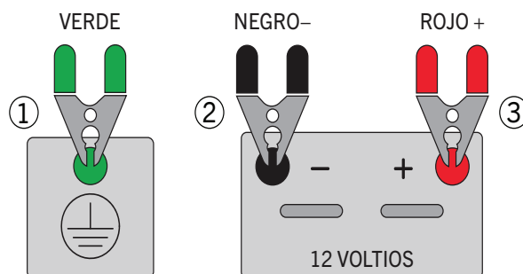
TIERRA / CONEXIÓN A TIERRA DEL CHASIS
